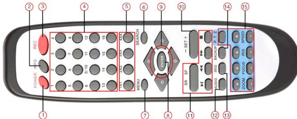
2-8. Ábra: Távirányító
