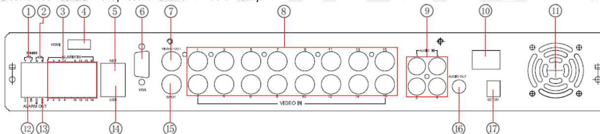
2-7. Ábra: A 16 csatornás készülék hátlapi csatlakozói
